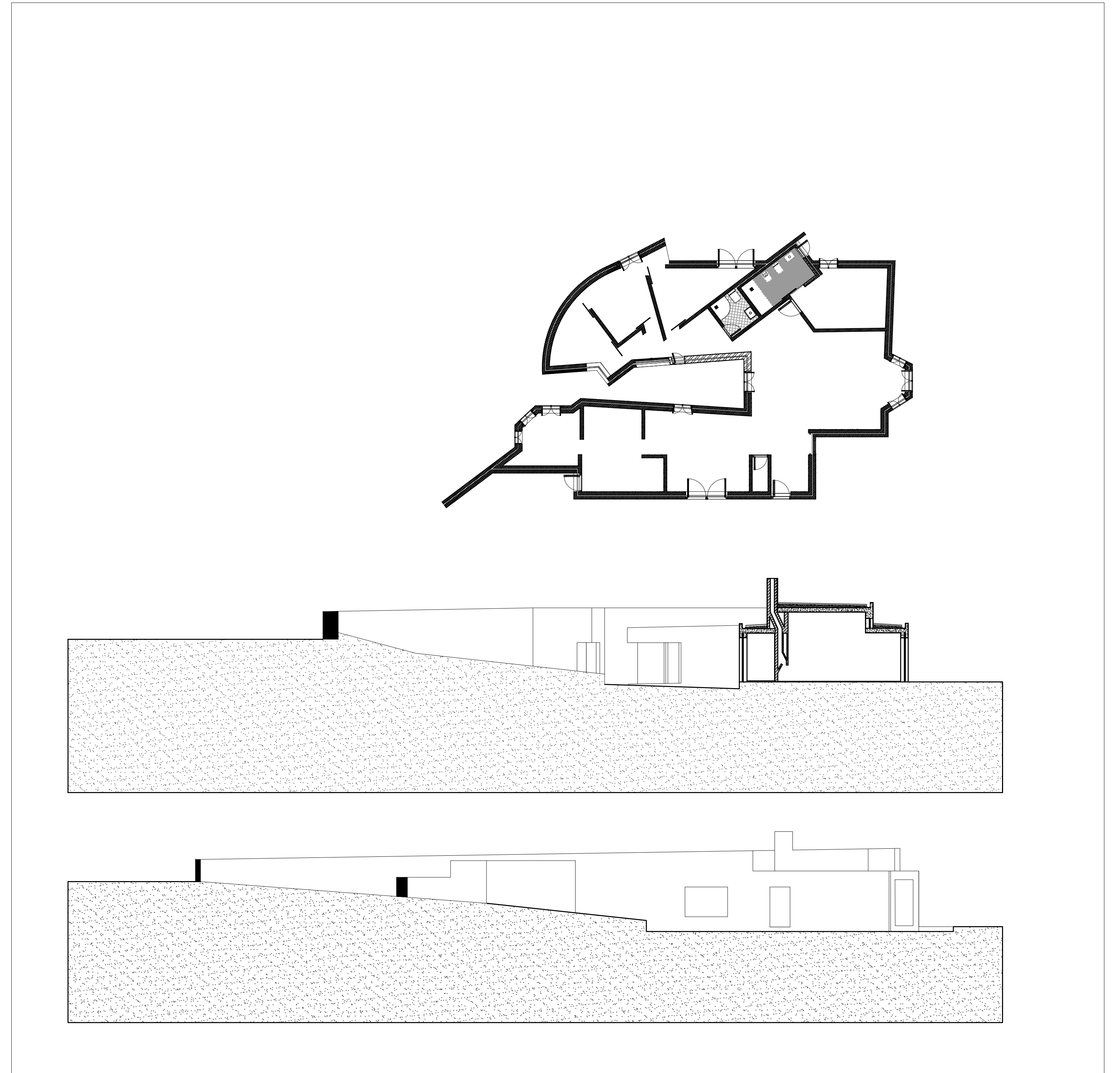
Planta + Alçados
